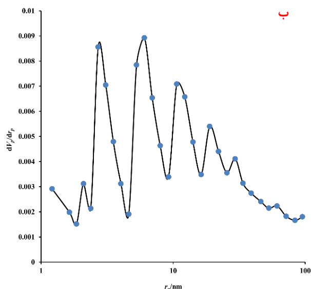
شکل ۵- نتایج آنالیز BET نانوکامپوزیت CTS/SBA-15 شامل: الف) ایزوترم جذب-واجذب نیتروژن؛ و ب) توزیع اندازه حفرات براساس روش BJH
