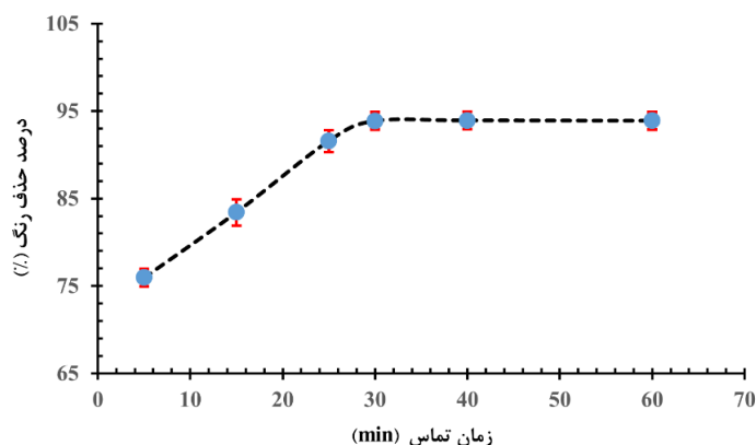
شکل ۹- اثر زمان تماس بر حذف متیل اورانژ توسط نانوجاذب CTS/SBA-15
