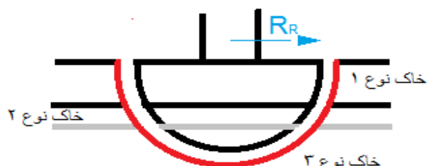
شکل ۲- شعاع صفحه ریشه و نیروهای برشی خاک
